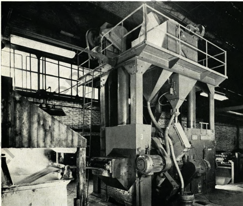
In dieser Anlage [Fabrikat Georg Fischer, Schaffhausen] werden jeden Monat weit über 1000 Tonnen Walzdraht mit dem im Werk Lippstadt erzeugten Drahtkorn UNIOSTRAHL mechanisch entzundert. Nach dem Bestrahlen durchlaufen die gereinigten Drähte das Kalkbad (im Vordergrund links).
