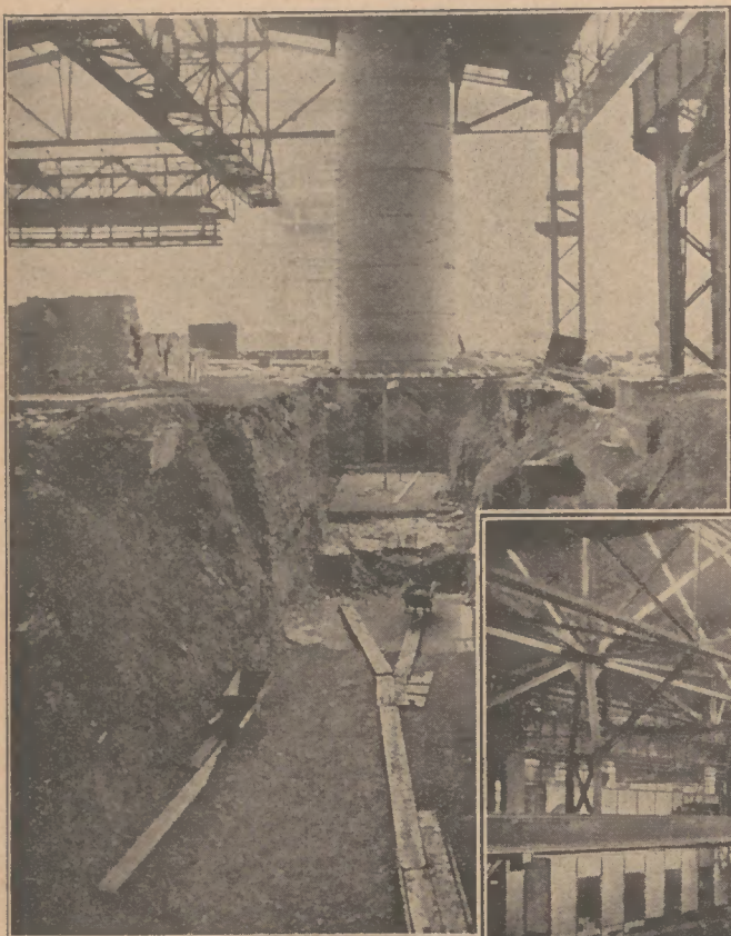
Abb. 13: Blick in die Baugrube für den Rauchkanal und auf den neuen Kamin. (18. 2. 26.)
