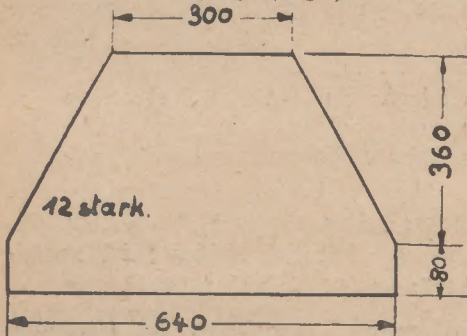
Das Knotenblech.
