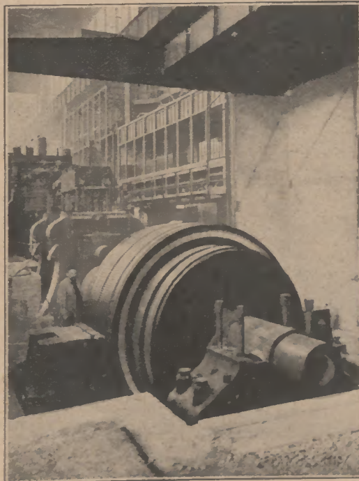
Abb. 11: Blick auf den Walzmotor der Vorstraße (18 000 PS). (18. 2. 26.)
