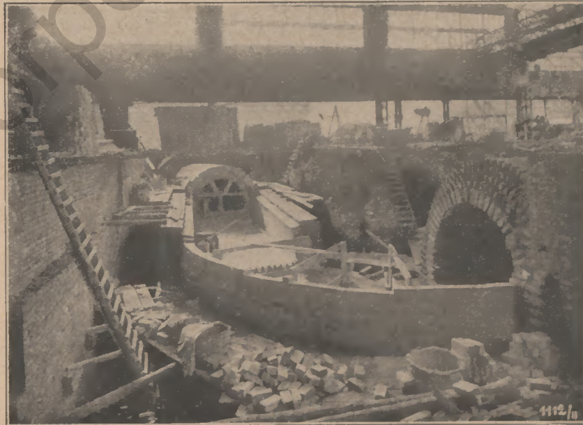
Abb. 12: Blick auf die Rauchkanäle hinter Ofen II. Unterer und vereiniger Kanal bis zum Kamin fertig. (13. 4. 26.)
