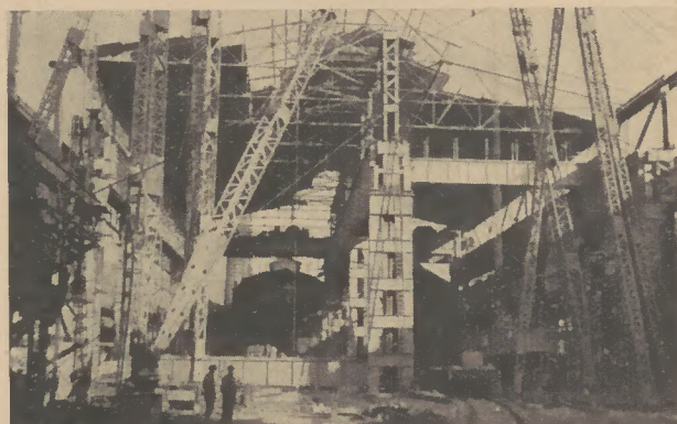
Halle im Aufbau — Zwei Gießkräne und ein Chargierkran sind schon gezogen
