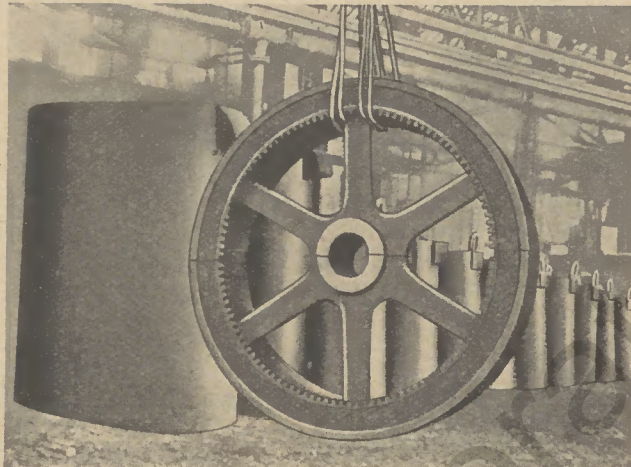
Rotillen verschiedener Größen sowie gußeisernes Polrad von 25 T. Gewicht
