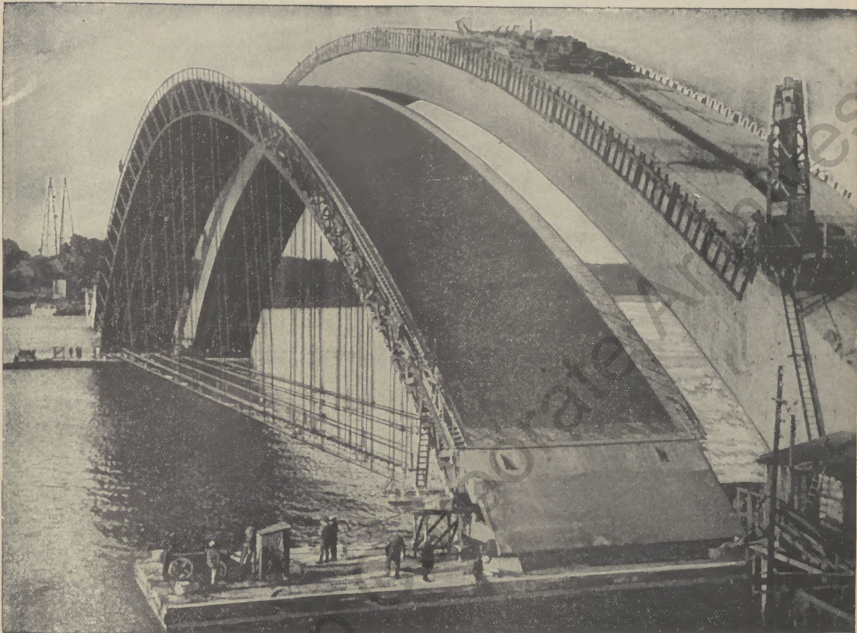
Abb. 1: Das Ausfahren des Lehrgerüsts aus einem fertiggestellten Eisenbetonbogen. (Aus einem Film des Deutschen Betonvereins)
