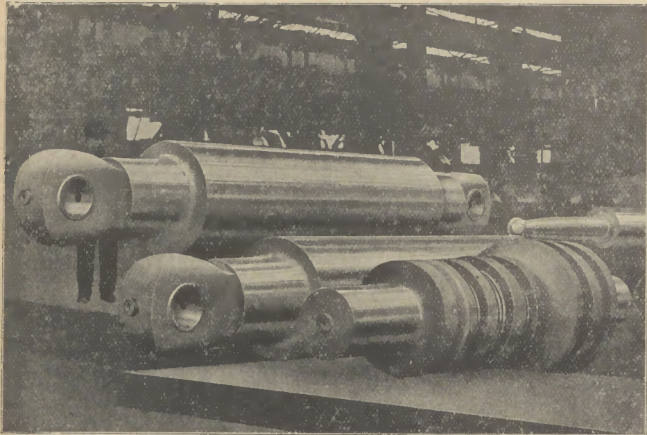
Eine Duo Blockwalze im Gewichte von 64 860 kg und eine schwere Mittelwalze im Gewichte von 25 800 kg
