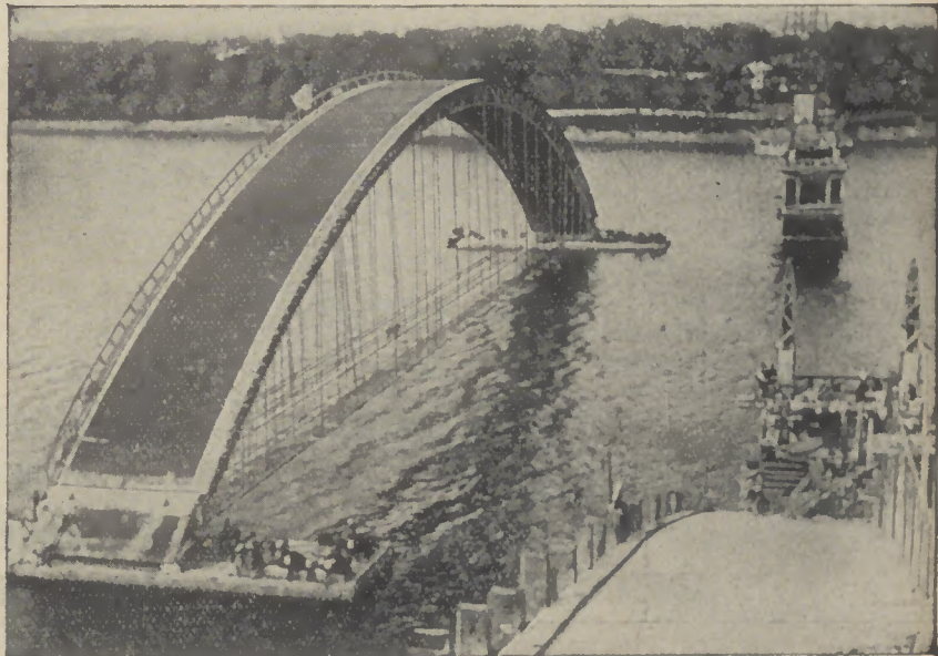
Abb. 3: Einfahren des Lehrgerüsts für einen neuen Eisenbetonbogen
