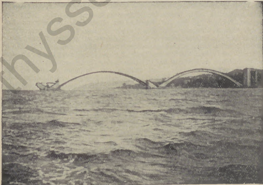
Abb. 2: Rechts: Ein fertiger Eisenbetonbogen; links: Das eingefahrene Lehrgerüst
