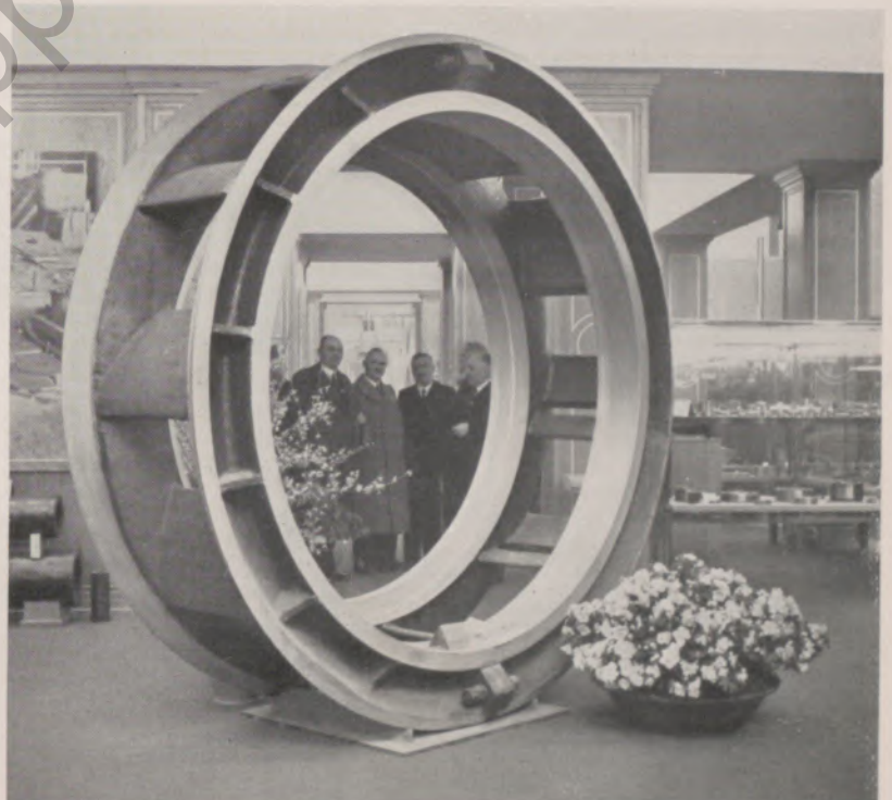
Traversenring für eine Wasserturbine aus EHW-Stahl
