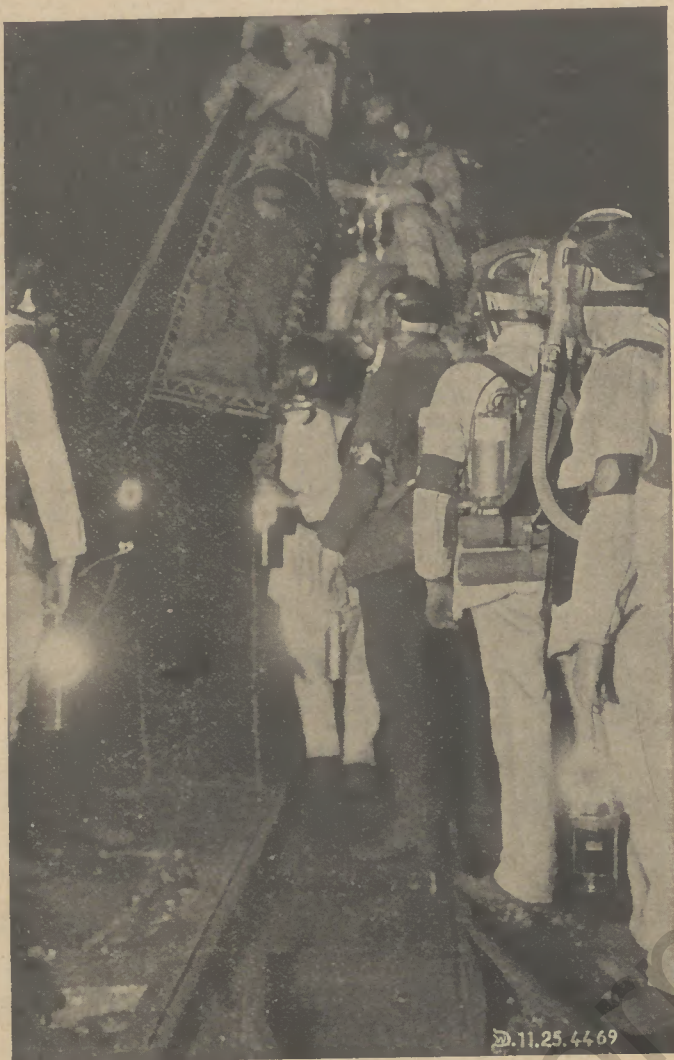
Verletzten-Transport mit Garczyks Steiltransportbahre des Draeger-Werks, Lübeck.
