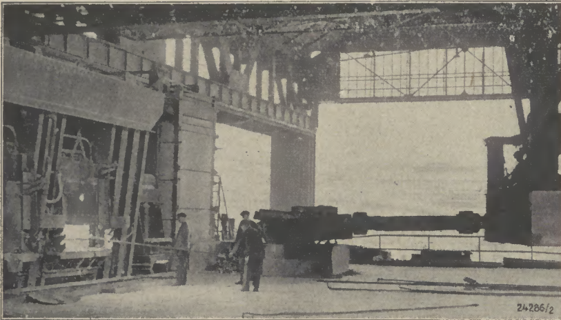
Neuer Salzofen im Martinstahlwerk der Hütte Ruhrort-Meiderich
