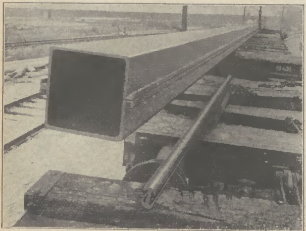
35 Meter lange Kastenbohle auf Waggons mit Schloß
