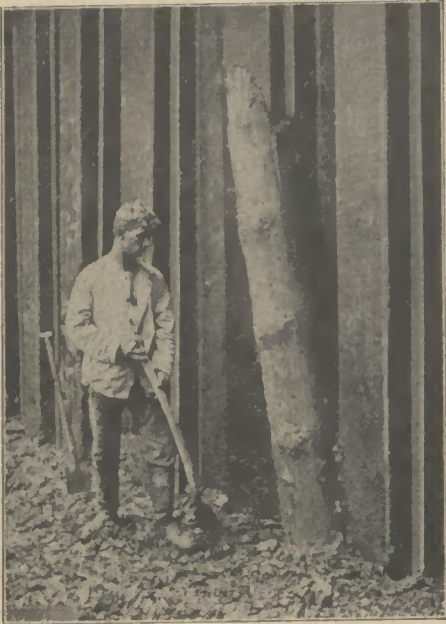
Von der Spundwand durchgerammter Pfahl (Drehpfahlfundament, Drehbrücke)
