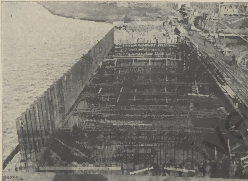
Westliche Spundwand am 31. Oktober 1929
