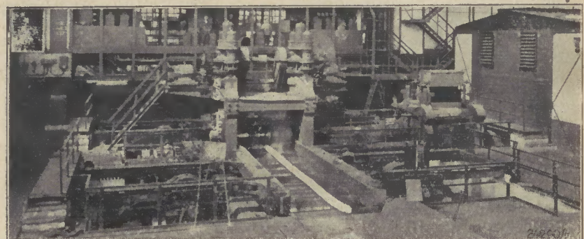
Walzenstraße im neuen Walzwerk IV der Dortmunder Union
