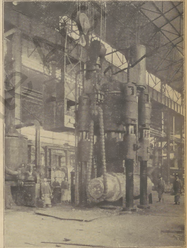
2000 tons-Schmiedepresse im Betrieb.
