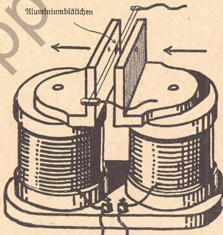
Abb. 1. Saitengalvanometer
