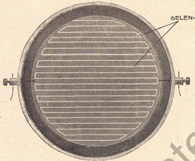
Abb. 2. Selenrundzelle durch Gravierung hergestellt
