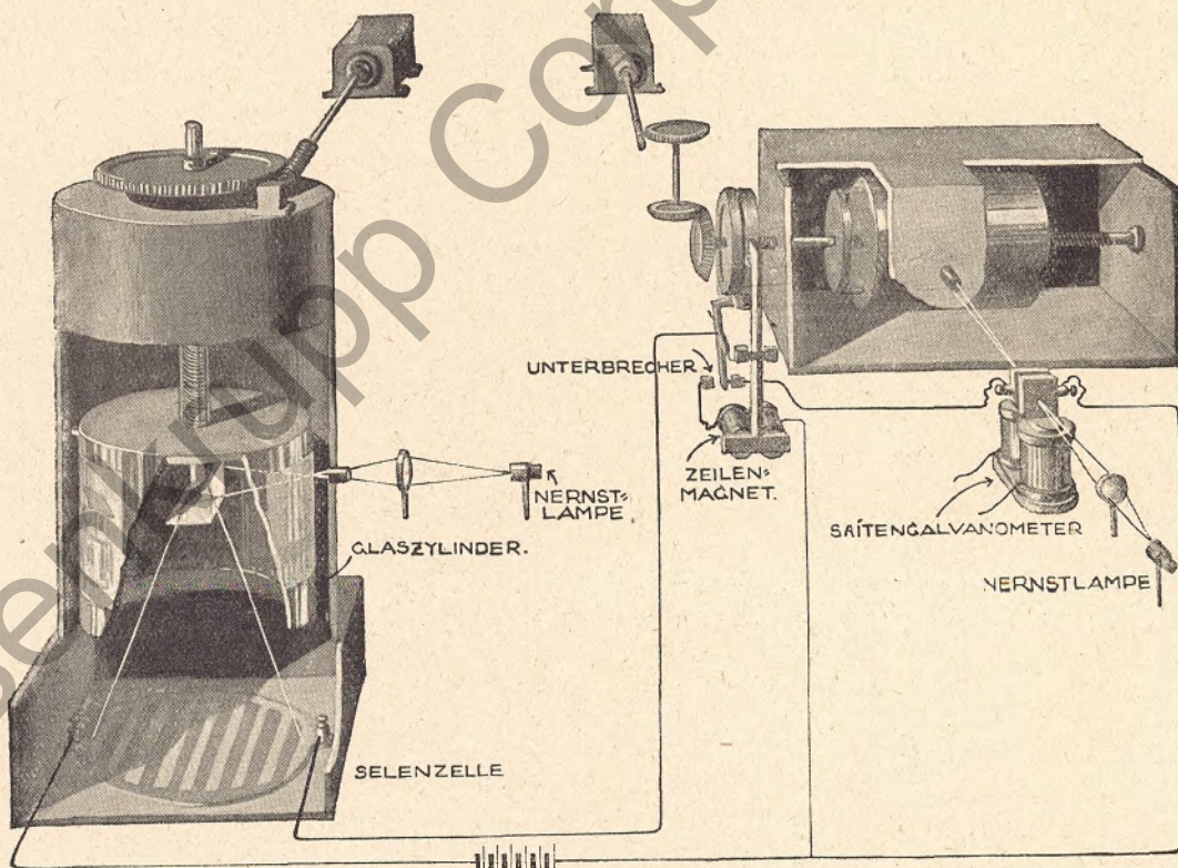
Abb. 3. Einrichtung für Selen-Bildtelegraphie nach Korn
