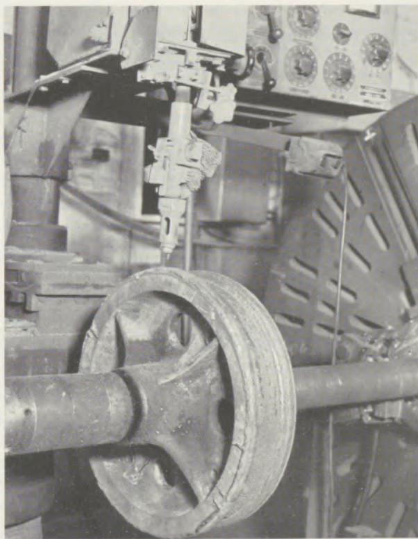
Waagrecht-Bohr- und Fräsmaschine; Spindel \varnothing 200 mm
