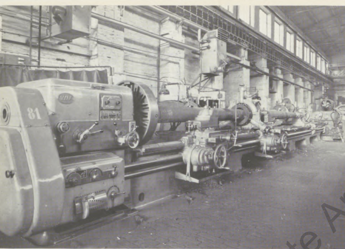
Spitzendrehbank, 350 mm Spitzenhöhe; 10000 mm Spitzenweite
