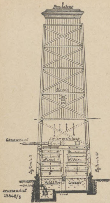
Zeichnerische Darstellung eines Kaminkühlers
