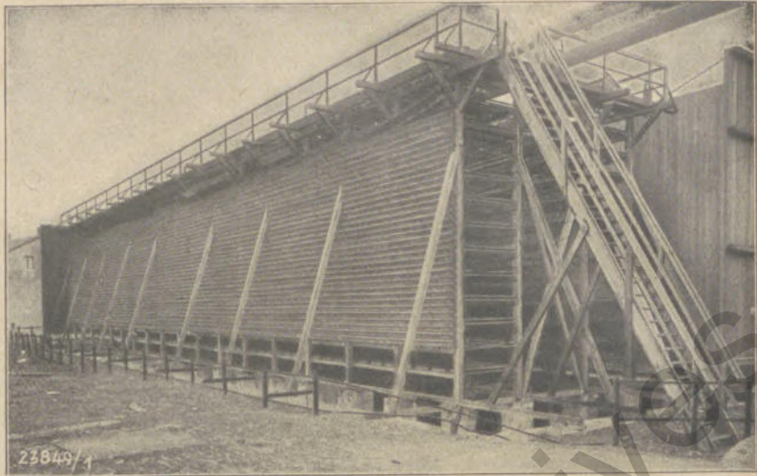
Gradierwerk einer Nebengewinnungsanlage
