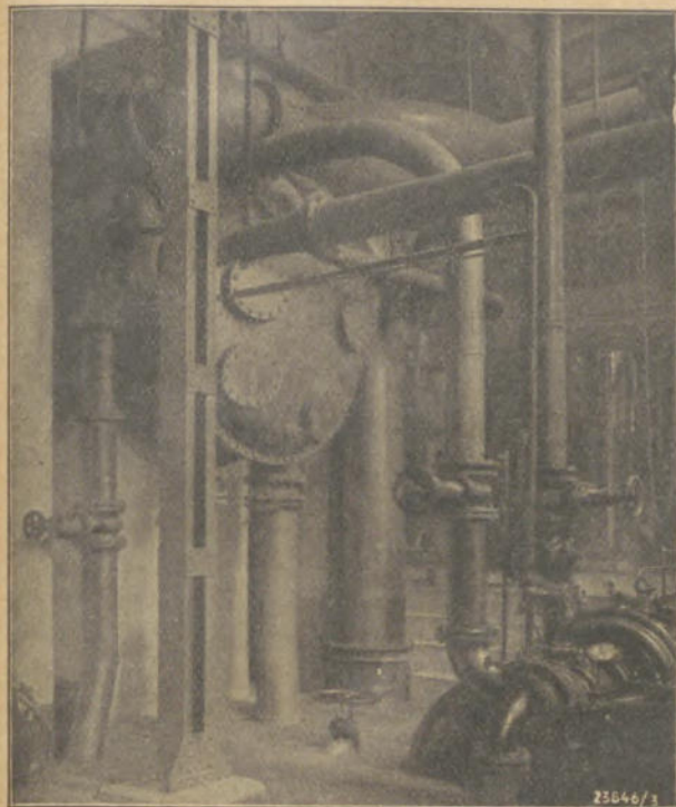
Kondensationsanlagen eines Turbo-Kompressors
