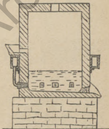
Abb. 10 Bessemer's feststehender Versuchsapparat
