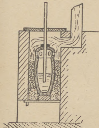
Abb. 9 Bessemer's erster Versuch
