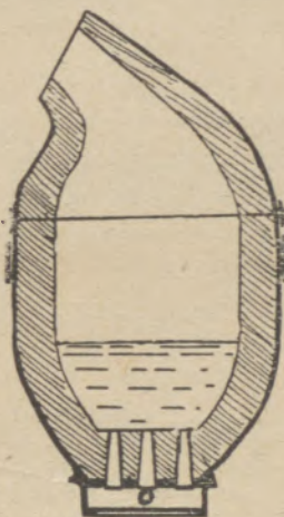
Abb. 11 Konverter des Stahlwerks Henry Bessemer & Co. in Sheffield 1859
