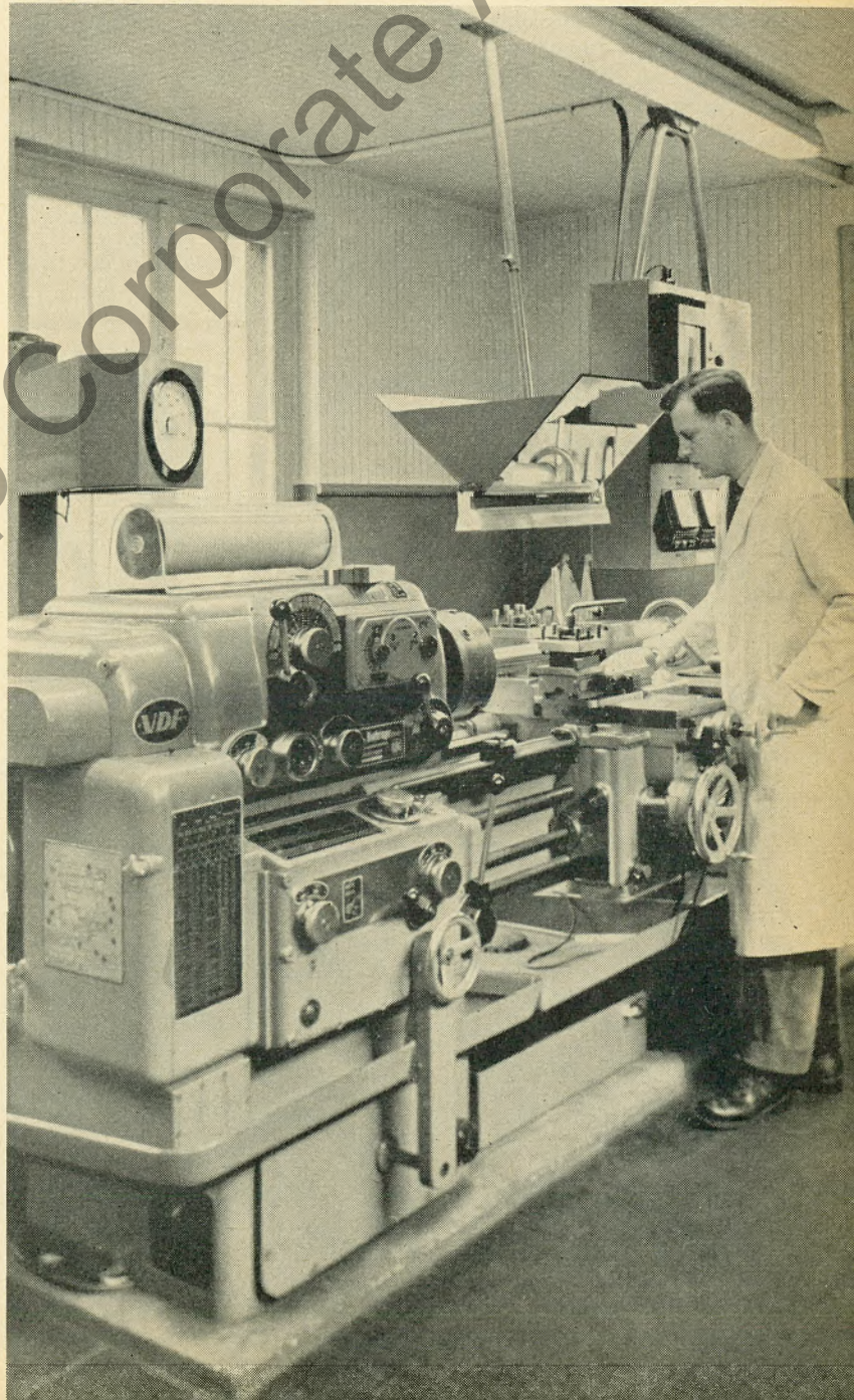
Prüfbank für Automatenstähle
