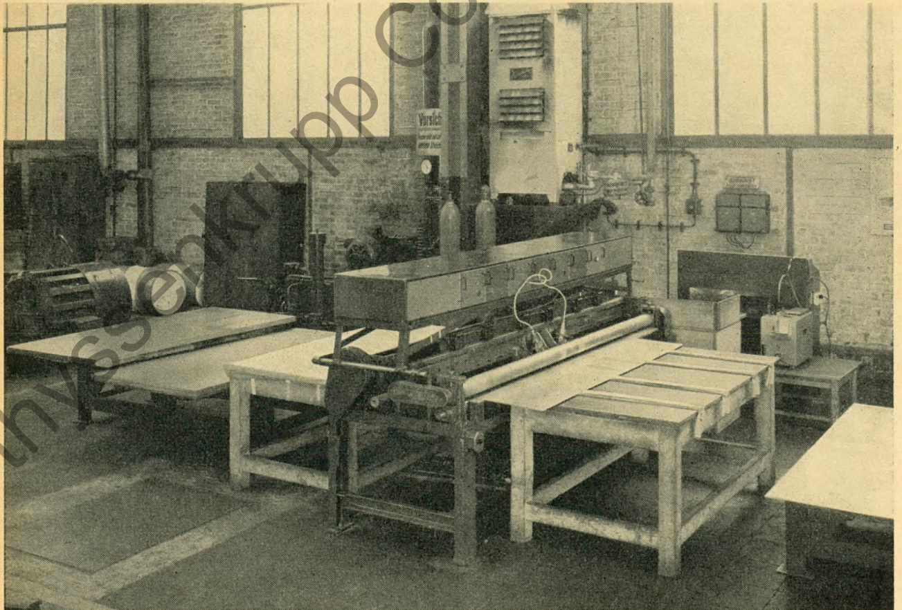
Ultraschallprüfanlage für Bleche
