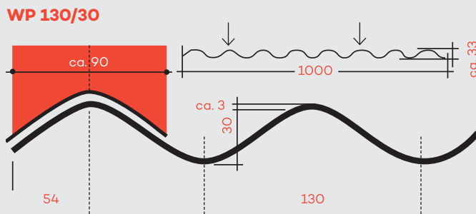
Querschnitt der PLEXIGLAS® Resist WP 130/30 (Maße in mm)
