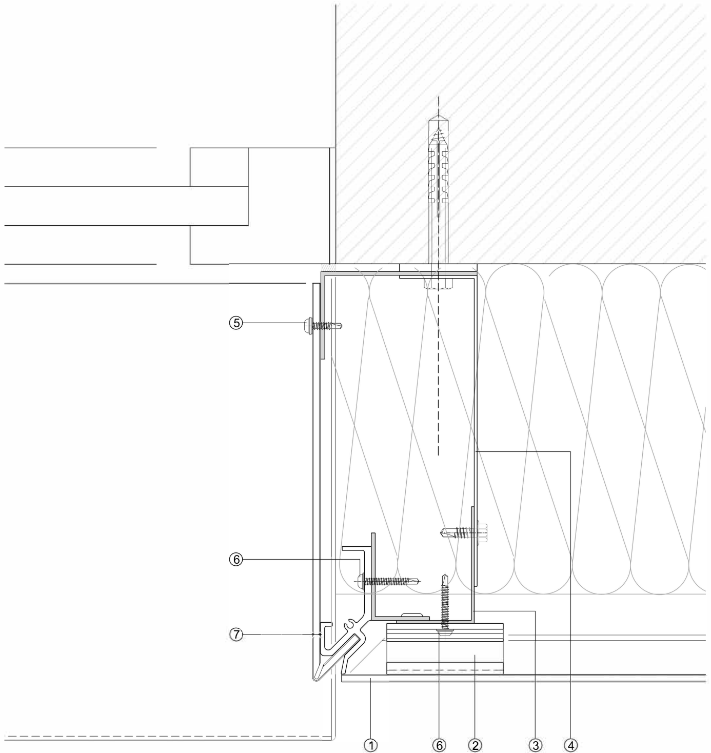
Abbildung zeigt eine mögliche Aluminium-Unterkonstruktion
