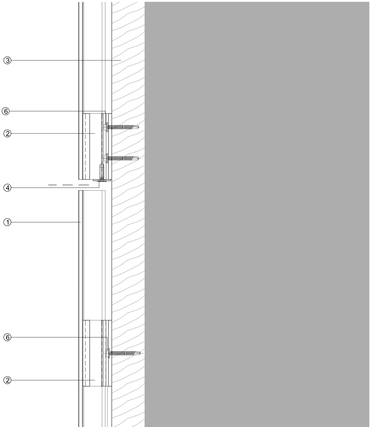
Abbildung zeigt eine mögliche Holz-Unterkonstruktion
