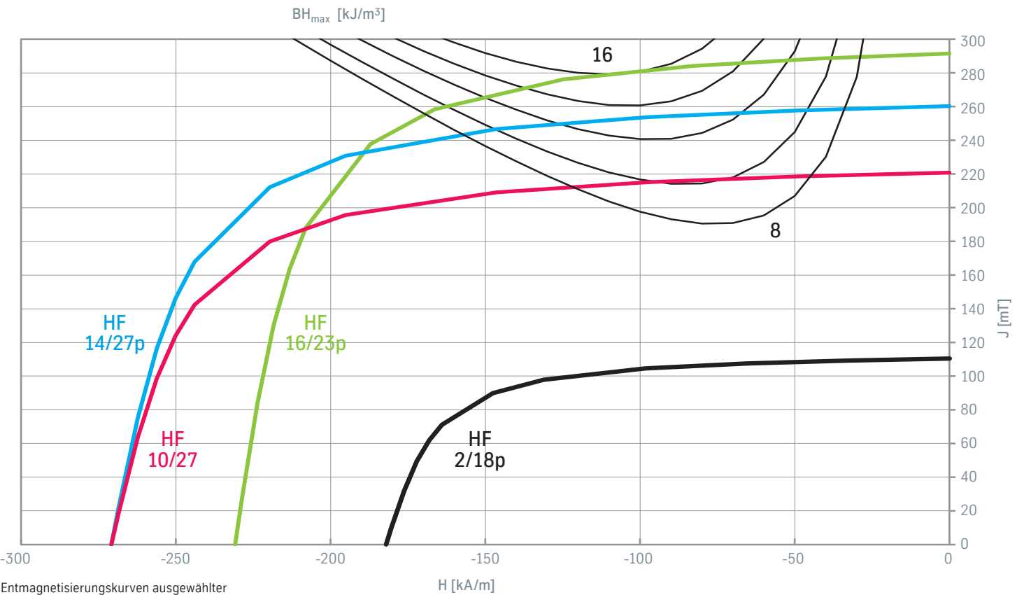
Entmagnetisierungskurven ausgewählter kunststoffgebundener Hartferrit-Magnete
