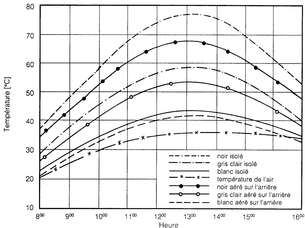
Courbe de température des plaques en PVC rigide en fonction de la couleur et de l'aération épaisseur des plaques 3-4 mm, influence de l'ensoleillement, température max. de l'air 36 °C
