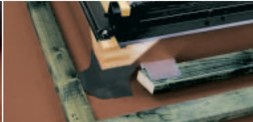
Verkleving met DELTA®-FLEXX BAND aan dakvenster.
