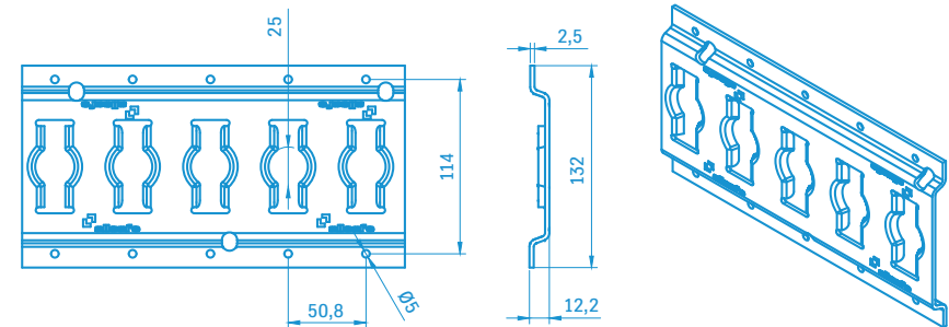
Combi-Zurrschiene allsafe 71219
