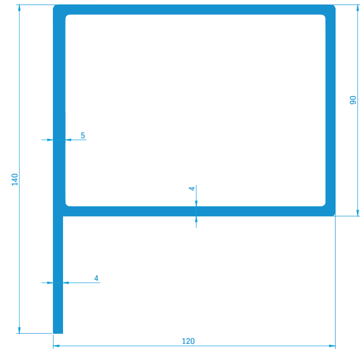
Eckprofil 80580 5,30 kg/m
