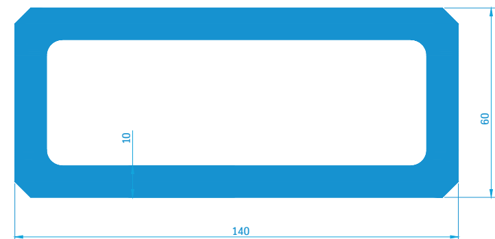
Vierkantrohr 80735 9,78 kg/m
