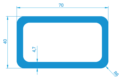
Vierkantrohr 40439 2,68 kg/m
