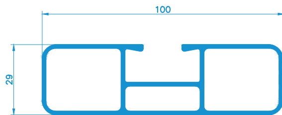
Seitenschutzprofil (roh/eloxiert) 70310 1,30 kg/m Passende Kappe zum Profil 70300
