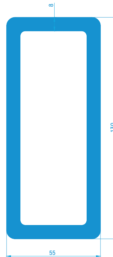
Vierkantrohr 80734 7,30 kg/m
