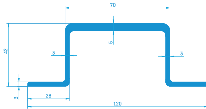
Hutprofil 80460 1,92 kg/m
