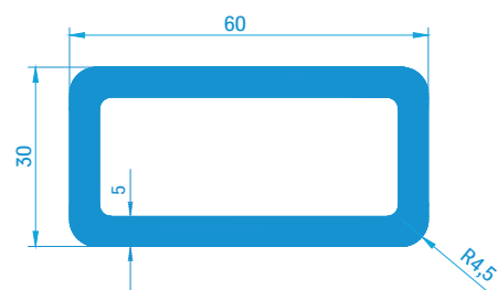
Vierkantrohr 40441 2,14 kg/m
