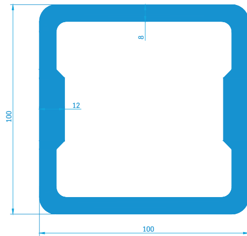
Vierkantrohr 80906 8,57 kg/m
