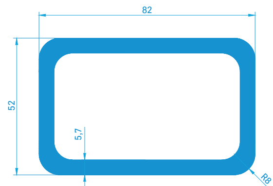
Vierkantrohr 40443 3,93 kg/m
