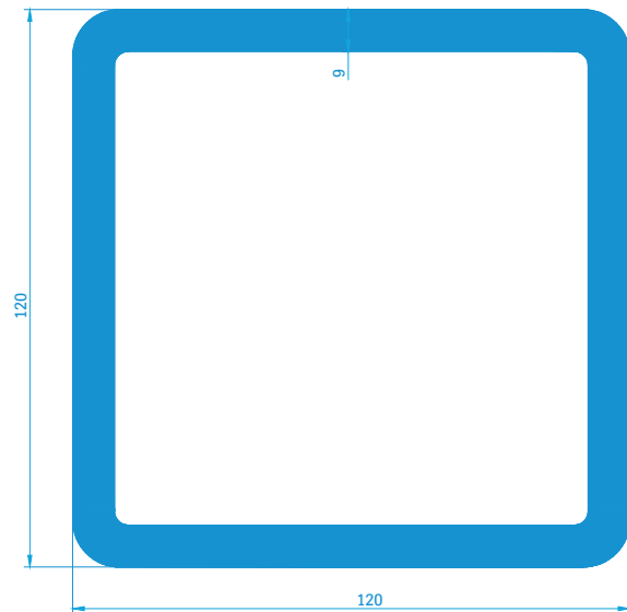
Vierkantrohr 80907 10,70 kg/m
