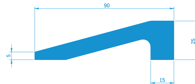
Anschlag Heckklappe 80953 3,00 kg/m
