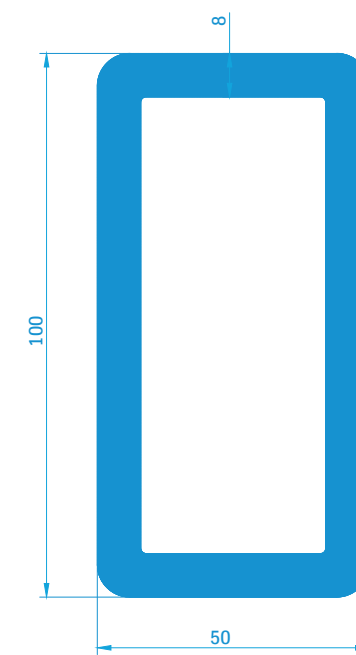
Vierkantrohr 80148 5,72 kg/m
