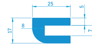
Führungprofil für Schieber 80119 0,75 kg/m
