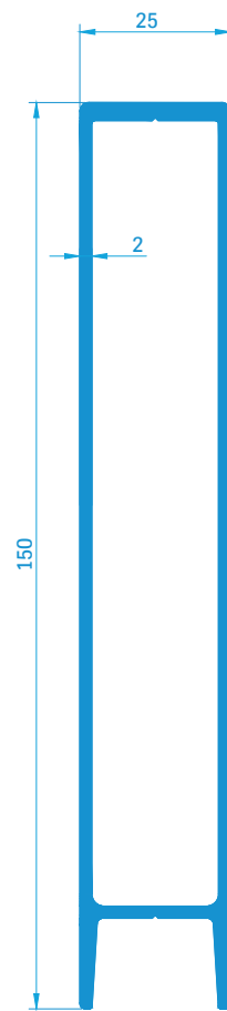
25105 1,90 kg/m
