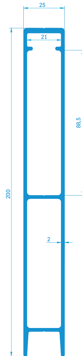
25083 2,65 kg/m
