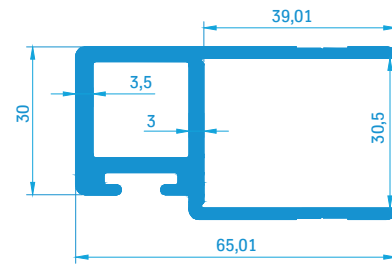
30423 1,56 kg/m
