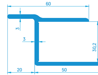
30907 0,97 kg/m
