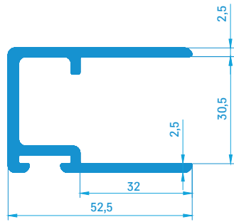
30642 1,05 kg/m
