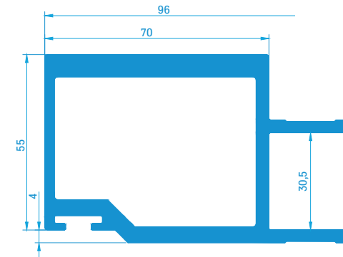
30819 3,68 kg/m
