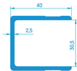
30381 0,75 kg/m
