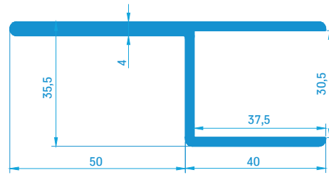
30113 1,29 kg/m
