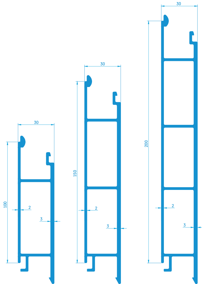
30813 1,87 kg/m
