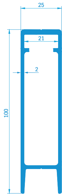
25092 1,27 kg/m
