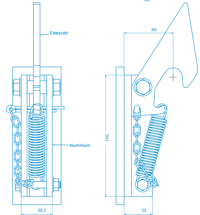
Hakenverschluss FZBZM50011
