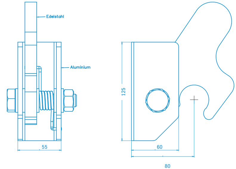
Hakenverschluss FZBZM50009
