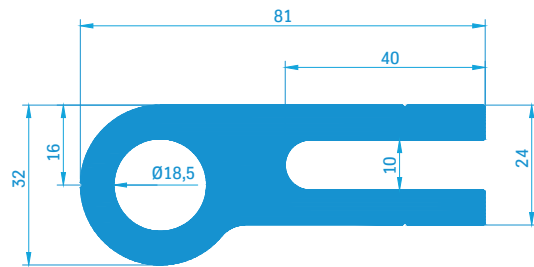
Scharnierprofil 80064 3,74 kg/m
