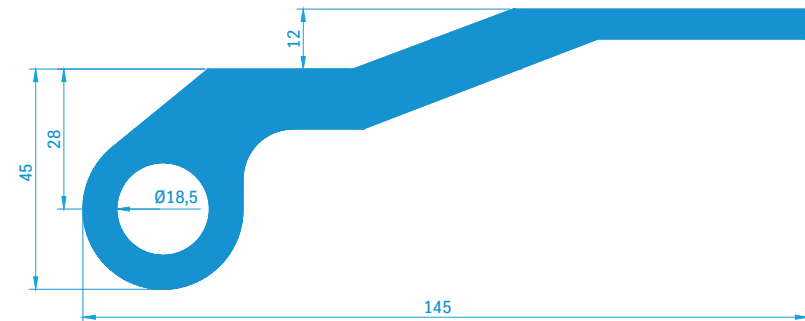
Scharnierprofil 80239 5,28 kg/m
