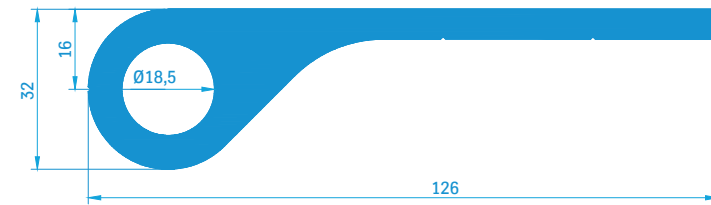
Scharnierprofil 80065 3,55 kg/m
