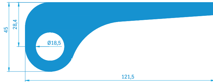
Scharnierprofil 80482 5,71 kg/m
