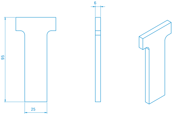
T - Stück 011 011
