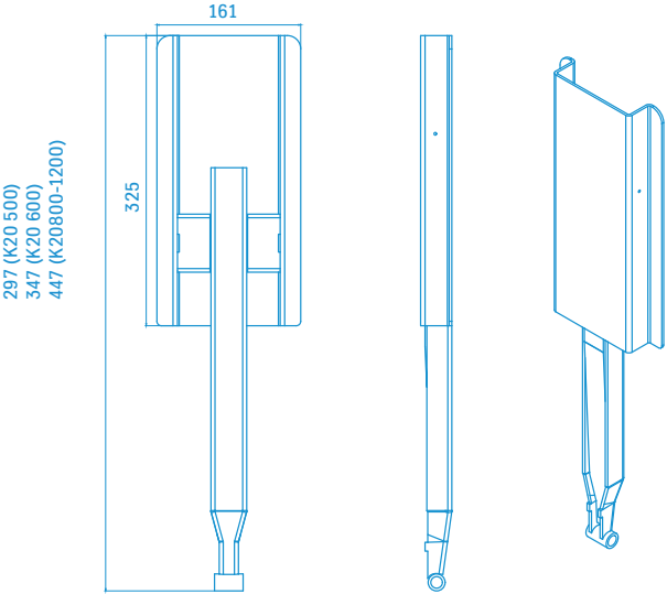
Kinnetop-Stativ
