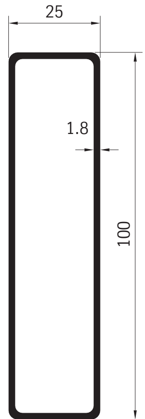
25021 1,17 kg/m
