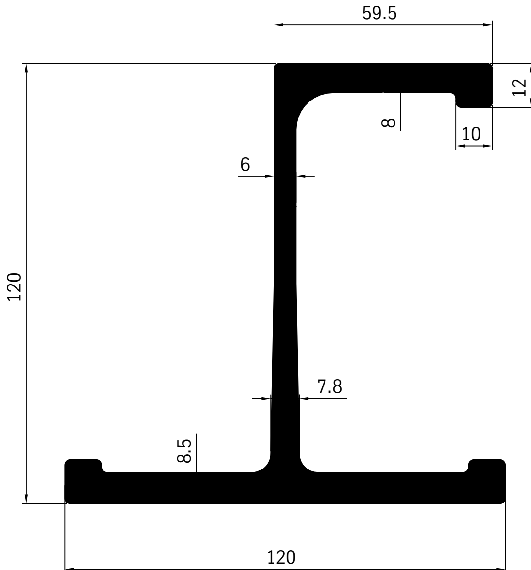
Querträgerprofil 80123 6,30 kg/m
