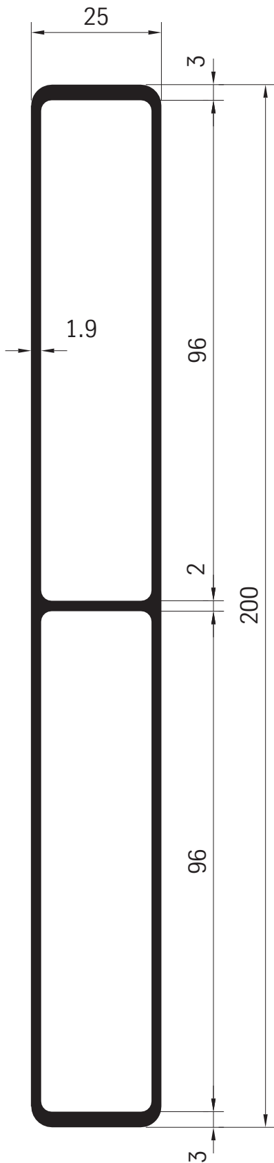
25121 2,49 kg/m
