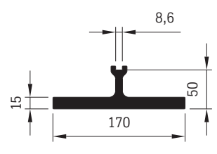
Trägerprofil 80458 8,40 kg/m
