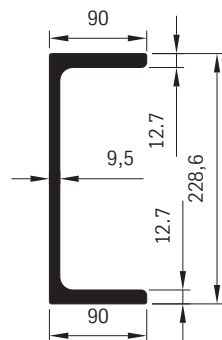
U-Profil 80230 11,88 kg/m
