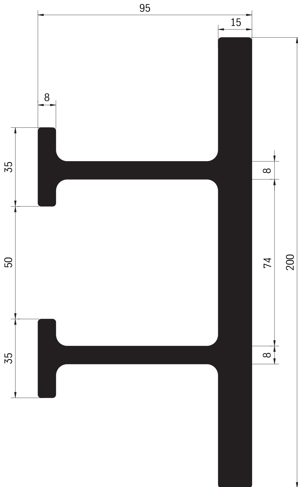
Trägerprofil 80143 12,80 kg/m
