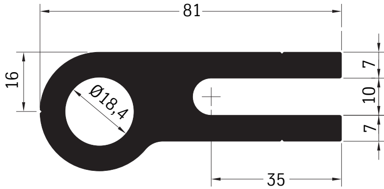
Scharnierprofil 80064 3,74 kg/m
