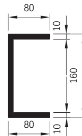
U-Profil 80160 8,20 kg/m
