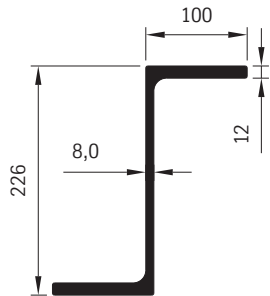
Z-Profil 80352 11,02 kg/m
