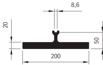
Trägerprofil 80457 12,22 kg/m
