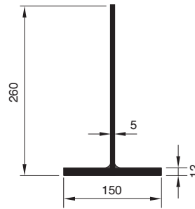
Trägerprofil 80260 8,38 kg/m
