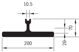
Trägerprofil 80456 12,96 kg/m
