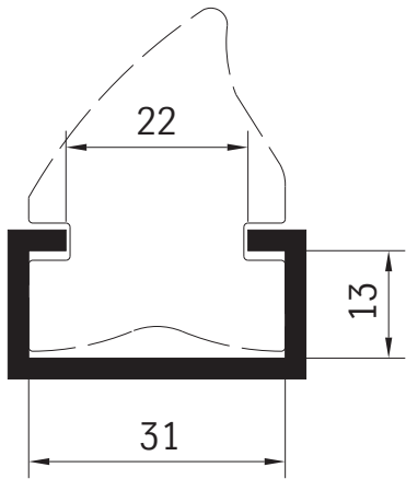
C-Schiene 80211 0,52 kg/m
